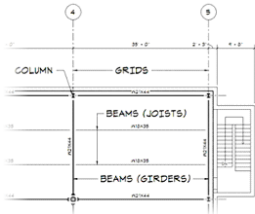
Plan med primärbalkar ( Girders ) och sekundärbalkar ( Joists ). Planritning med noteringar.
