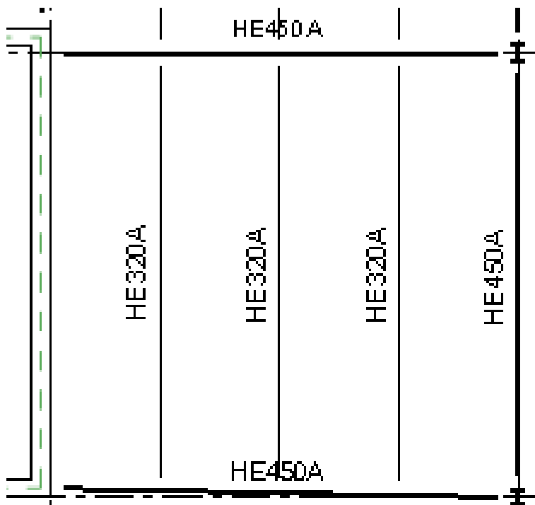
Oregelbunden och regelbunden balkdragnig i en planvy. HE450A primärbalkar ansluter pelare och konstruktionsvägg och sekundärbalkar HE320A stödjer i spannet.
